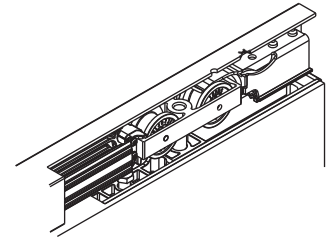
HAWA-Junior 80/B
